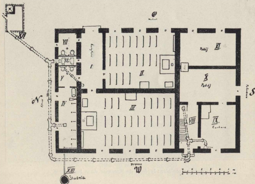
Ecole rurale à 2 classes, avec bains et canalisation.
