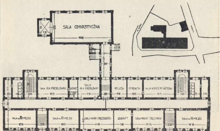
Ecole primaire Sienkiewicz, à Lwów. Façade, plan du rez-de-chaussée, plan de situation.
