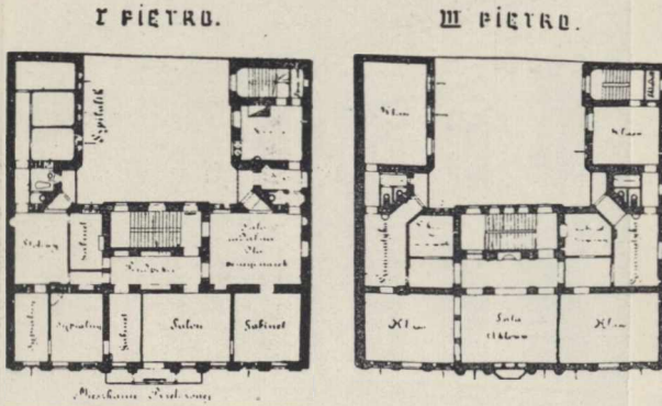
Ecole secondaire de filles (M-me Tolwińska, Varsovie). Plan du I. et III. étage.
