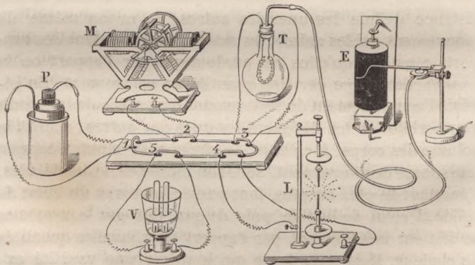
Fig. 1. — Montrant la transformation de l'électricité d'une pile, en travail mécanique, en chaleur, en lumière et en action chimique.
