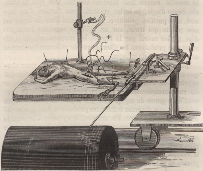
Fig. 3. — Myographe de Marey.
