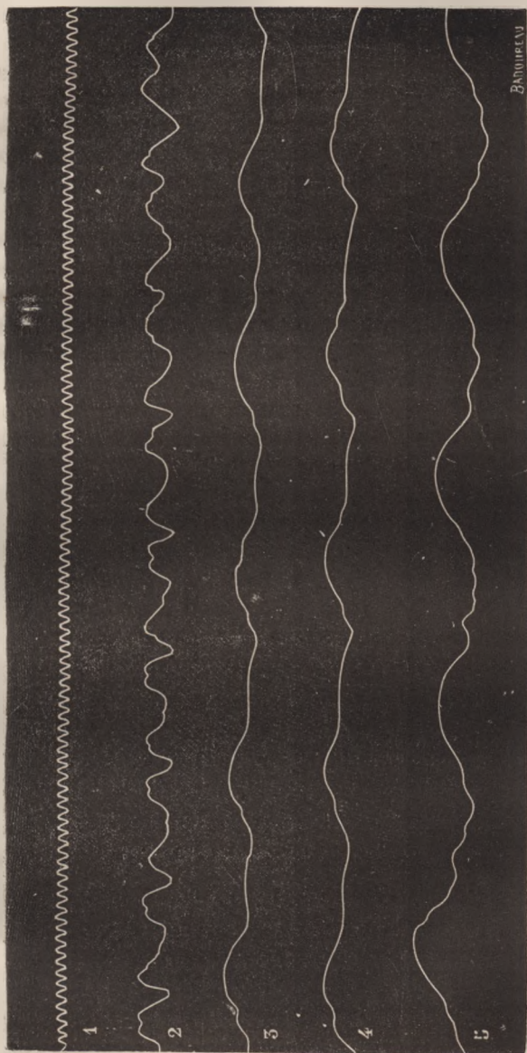
Fig. 113. — Ligne 1, tracé du diapason chronographe, où vibrations à la seconde. — Ligne 2, oscillations verticales du canard sauvage pendant le vol. — Ligne 3, oscillations du busard. — Ligne 4, chouette effraie. — Ligne 5, base.
