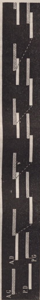
Fig. 66. Transition du trot au galop.
