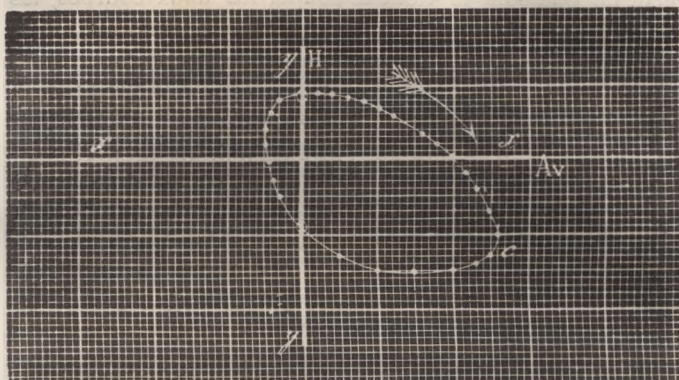
Fig. 107. — Construite d'après les courbes précédentes. — Une flèche indique le sens du mouvement. — L'écartement des points exprime la vitesse du mouvement de l'aile dans les divers instants de son parcours.
