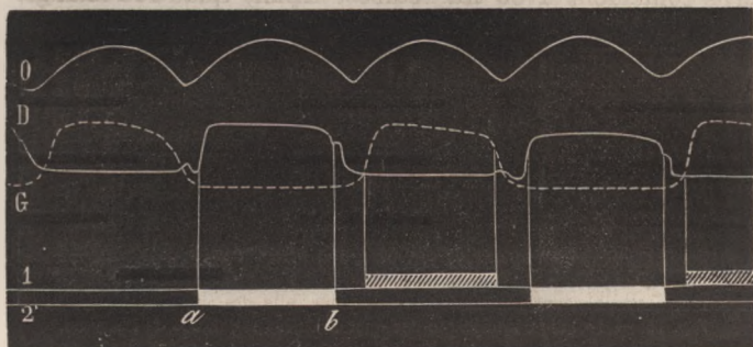
Fig. 34. — Notation d'un tracé de la course de l'homme.
