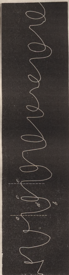
Fig. 115. — Trace simultanée des deux oscillations qu'une buse exécute en volant.
