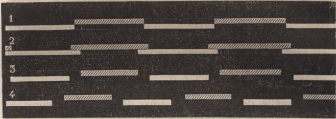
Fig. 33. — Notation synoptique des quatre allures régulières de l'homme.
