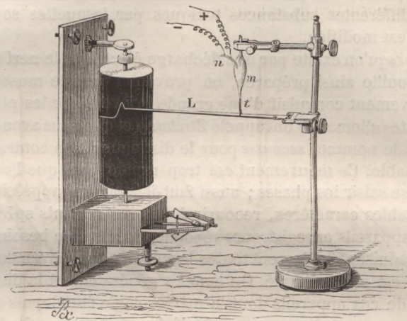
Fig. 2. — Description théorique du myographe.
