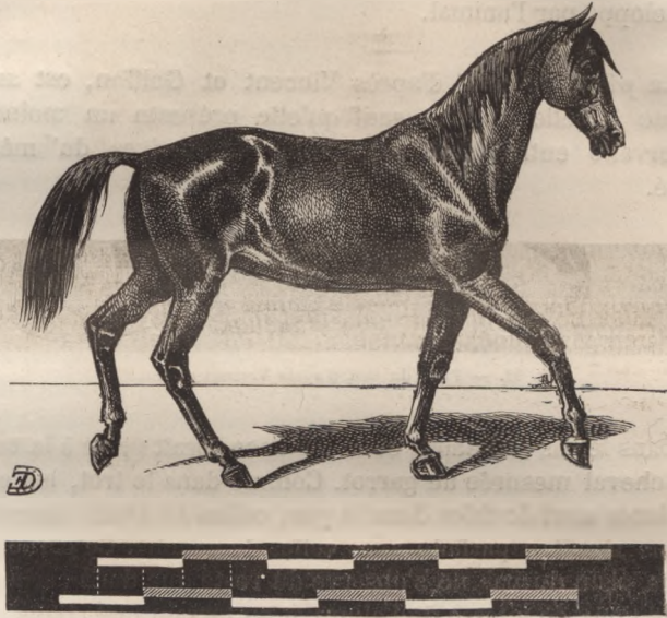
Fig. 54. — Représentation du cheval au pas.
