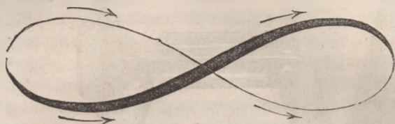
Fig. 86. — Trajectoire de l'aile.
