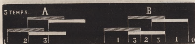
Fig. 56. — Galop à trois temps. A, indication des trois temps; B, indication du nombre des pieds qui forment l'appui du corps à chaque instant du galop à trois temps.
