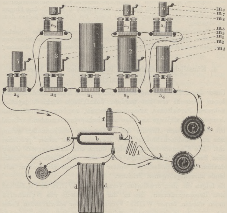
Helmholtz' Stimmgabelapparat zur Vokalsynthese.
