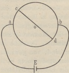
Schema des Fleischlschen Orthorheonom.
