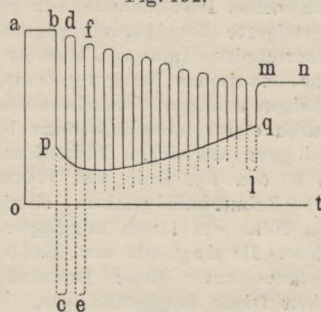
Die negative Schwankung bei Beobachtung mit dem Galvanometer.
