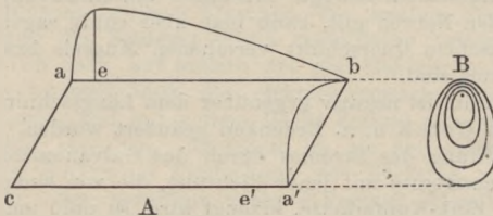
Spannungsverteilung am regelmäßigen Muskelrhombus.
