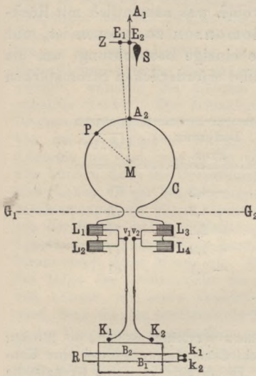
Anordnung von Einthoven.
