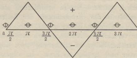
Stromverlauf bei Verwendung des Orthorheonom.
