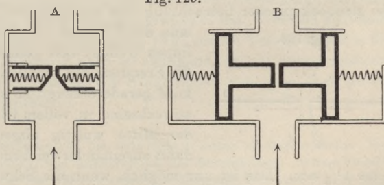
Zwei Polsterpfeifen (Gegenschlagpfeifen), nach Ewald. Der Pfeil gibt die Anblaserichtung an. Pfeife A kann nur in der vorgezeichneten Richtung angeblasen werden, B auch in der umgekehrten.
