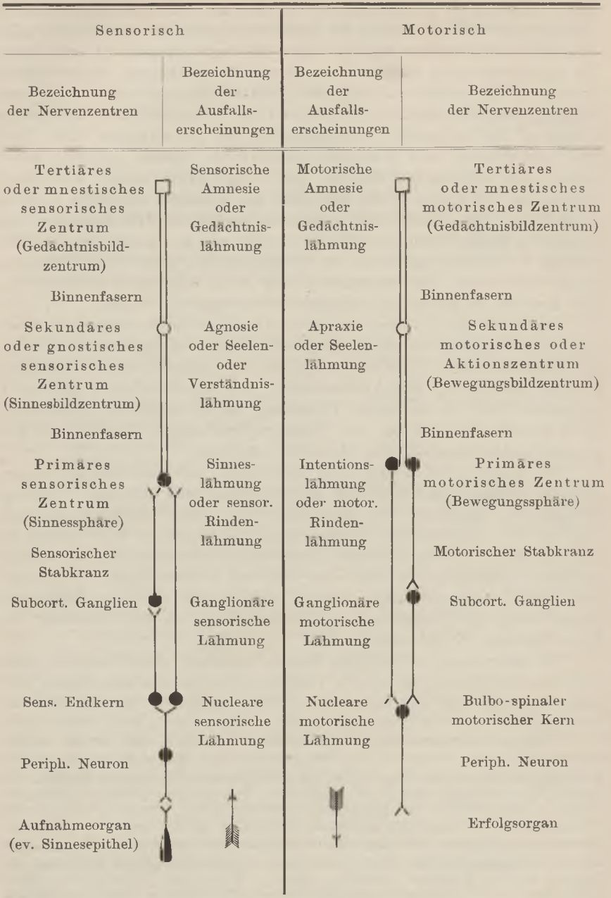
Schema I 1) .
