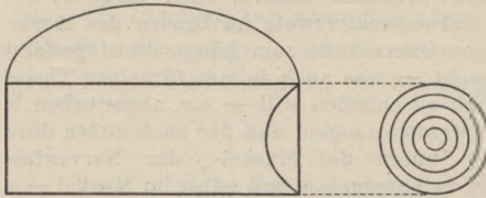
Spannungsverteilung am geraden Muskelprisma.
