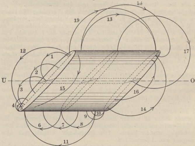
Strome am regelmäßigen Muskelrhombus.
