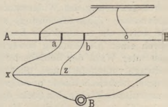
Schema der Abstufung linearer Stromschwankungen.
