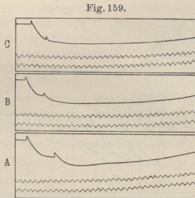
Aktionsströme bei zwei kurz aufeinander folgenden Reizen. Die Stimmgabel macht 500 ganze Schwingungen. Temperatur 4° C.
