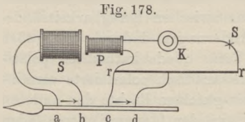
Grünhagens Versuch über Etablierung des Anelektrotonus.
