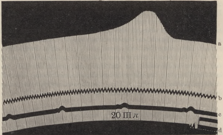
Monophasischer Aktionsstrom des Hechtfactorius nach Garten.
