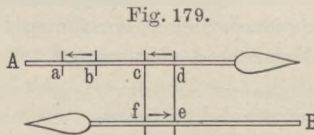
Schema zu Pflügers Versuch über Etablierung des Elektrotonus. [Hermann, Handbuch 2 (1), 163.]
