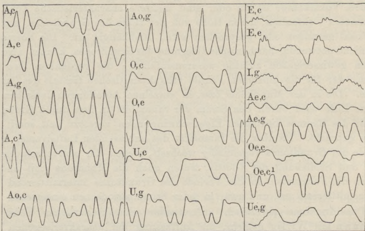
Vokalkurven nach L. Hermann.
