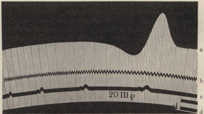
Diphasischer Aktionsstrom des Hechtfactorius nach Garten.
