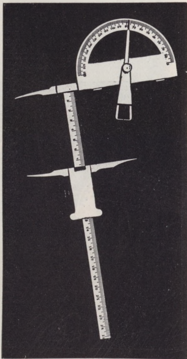
Fig. 274. Ansteckgoniometer am Gleitzirkel zur Messung der Gesichtswinkel.
