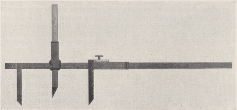
Fig. 271. Koordinatenzirkel.
