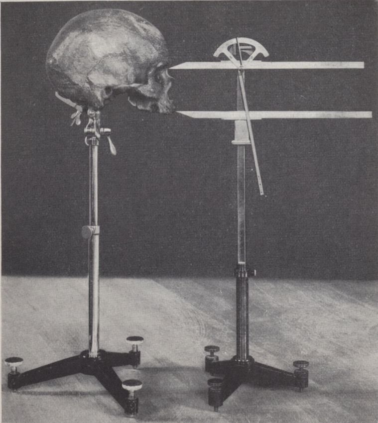
Fig. 272. Stativgoniometer mit Schädel auf Röhrenkraniochor.
