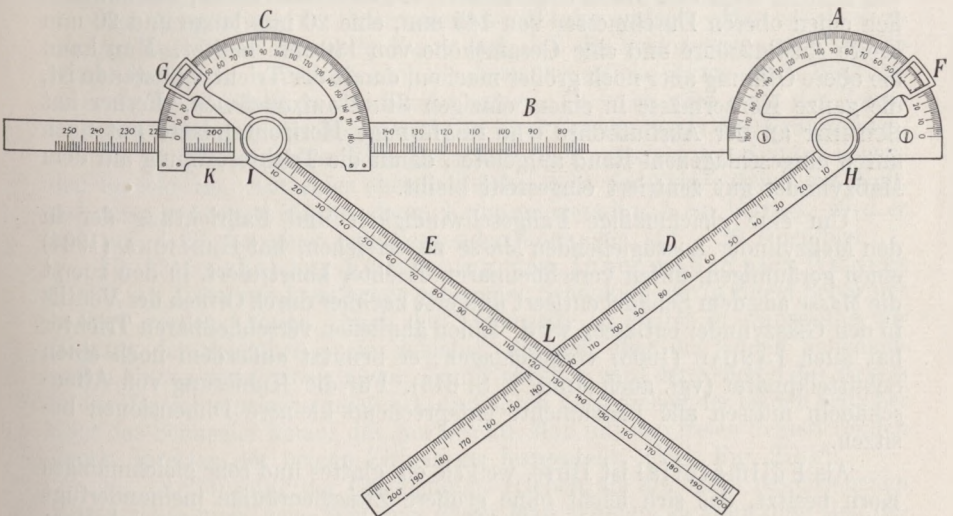
Fig. 277. Trigonometer. (Nach Fürst.)
