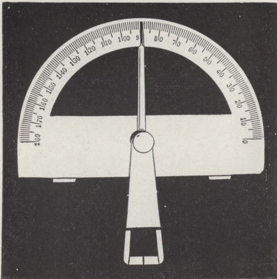
Fig. 273. Ansteckgoniometer. (Nach MOLLISON.)
