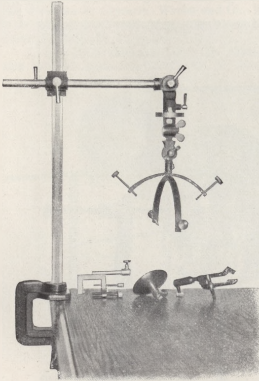
Fig. 283. Osteophor-Projektometer. (Nach STOLYUWO.) Der Bogenhalter ist angeschraubt, drei andere Halter liegen auf der Zeichenplatte.
